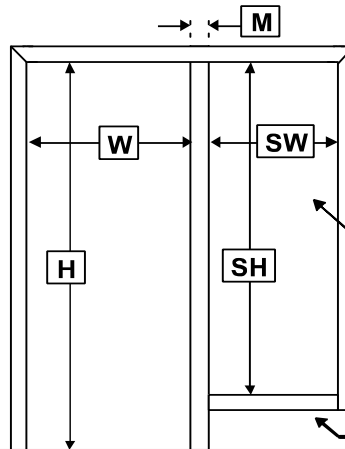
DOOR FRAME / SIDELIGHT
